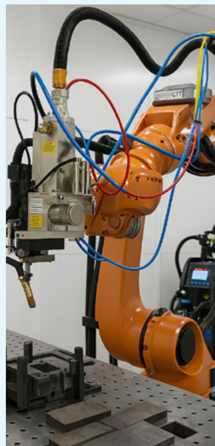
Robot equipado con tecnología de fabricación avanzada WAAM con aporte de hilo
